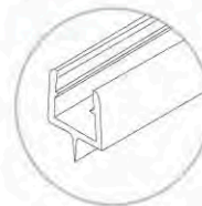
BRK 207 Botaguas lengüeta central suave para cristal de 8 a 10 mm.
