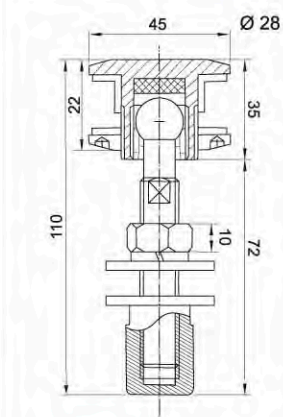
BRK Z01A Conector para araña soldable a estructura metálica plana o curva.
