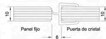
BRK 207 Botaguas lengüeta central suave para cristal de 8 a 10 mm.
